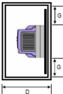
Размеры невентилируемого металлического шкафа (мм)
